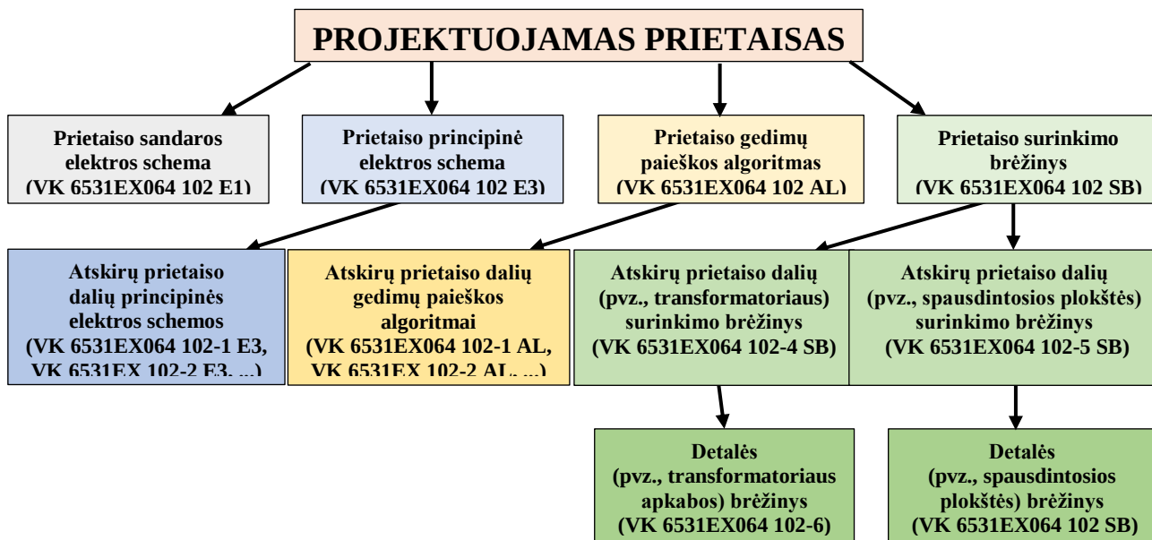
4.2 pav. Įvairių konstrukcijos dokumentų numerių sudarymo schema pagal suteiktą pagrindinį brėžinio numerį
